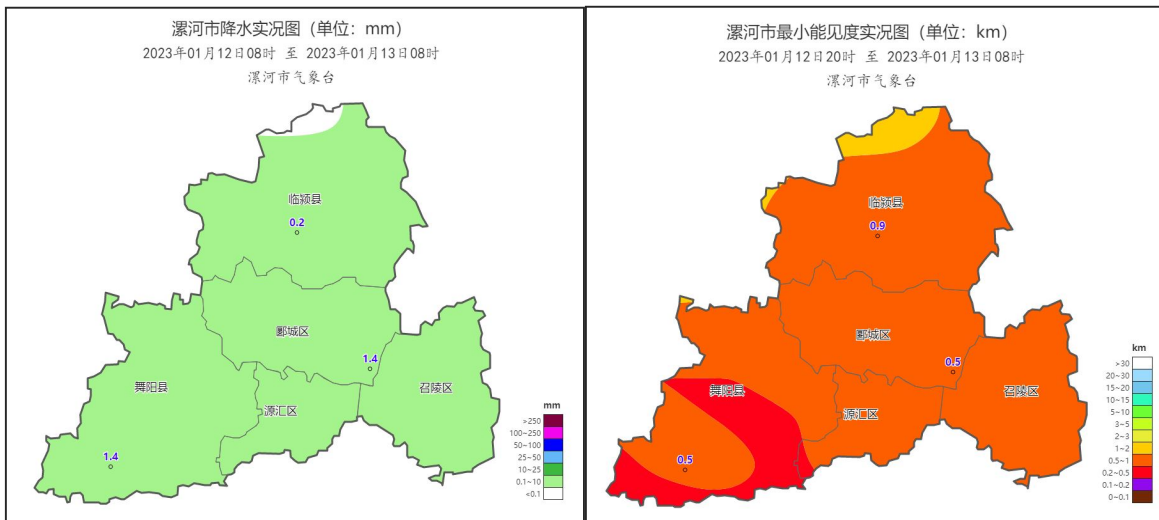
图 1 1 月 12 日 08 时至 13 日 08 时漯河市降水实况 (单位: mm) 和 1 月 12 日 20 时至 13 日 08 时漯河市最小能见度实况 (单位: km)
