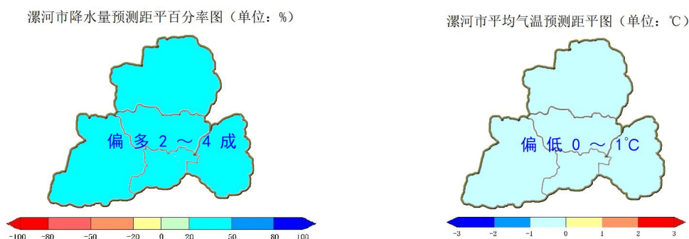
图 1 漯河市 2022 年 9-10 月降水距平百分率预测图(左)和气温距平预测图(右)
